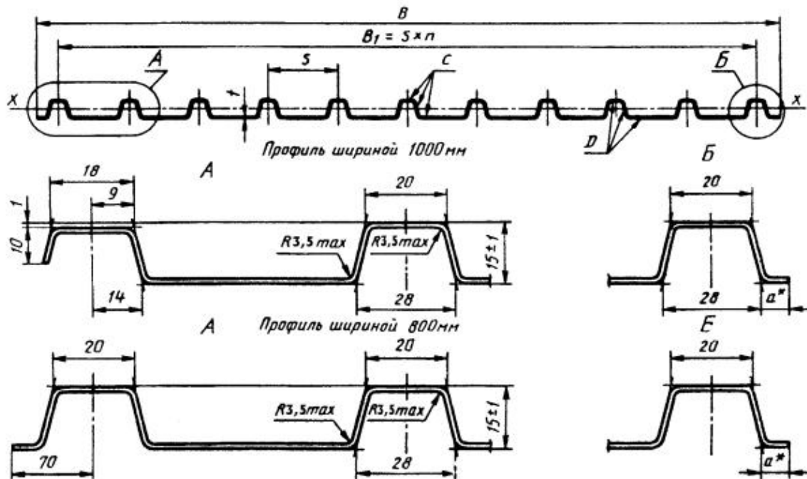
Рисунок 8 - Профилированный лист типа С высотой 15 мм
