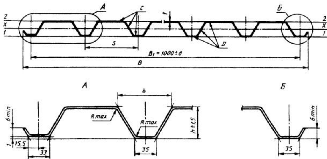
Рисунок 9 - Профилированный лист типа С высотой 21 и 44 мм
