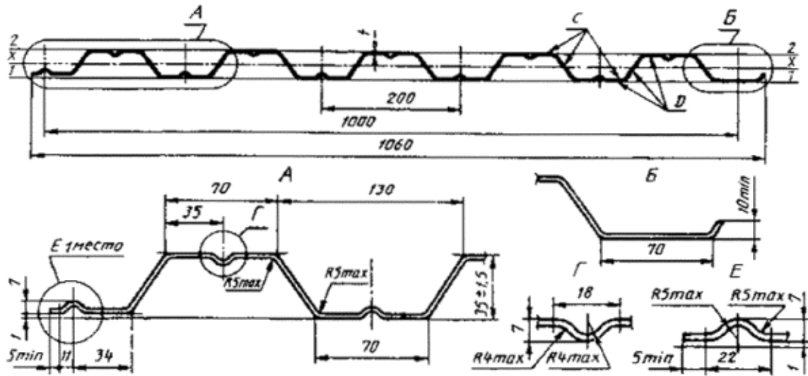
Рисунок 5 - Профилированный лист типа НС высотой 35 мм
